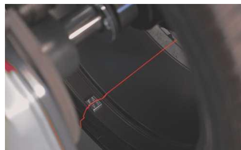
Laserový ukazatel pozice nalep. závaží
